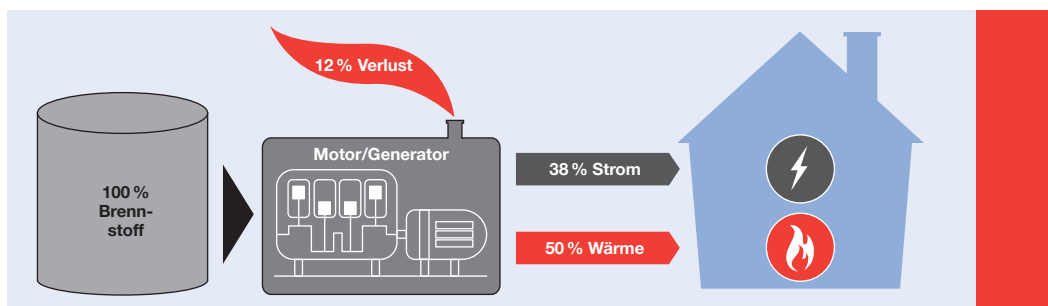
06 Schema Kraft-Wärme-Kopplung
