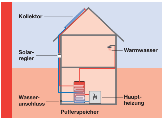
03 Funktionsaufbau solarthermische Anlage
