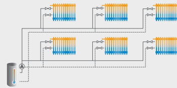
Hydraulisch abgegliche Anlage
