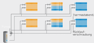
Hydraulisch nicht abgegliche Anlage
