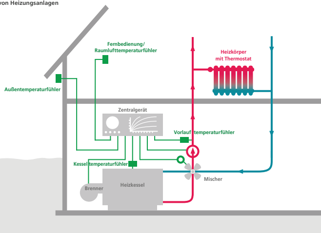
Regelung von Heizungsanlagen
