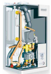
▲ Kompakte Heizungen und Brennwerttechnik haben sich durchgesetzt. Oft reicht heute für den Wärmebedarf eines gesamten Einfamilienhauses schon ein kompaktes, wandmontiertes Gerät.
