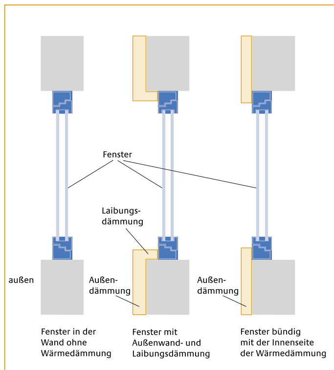
Einbausituation des Fensters
