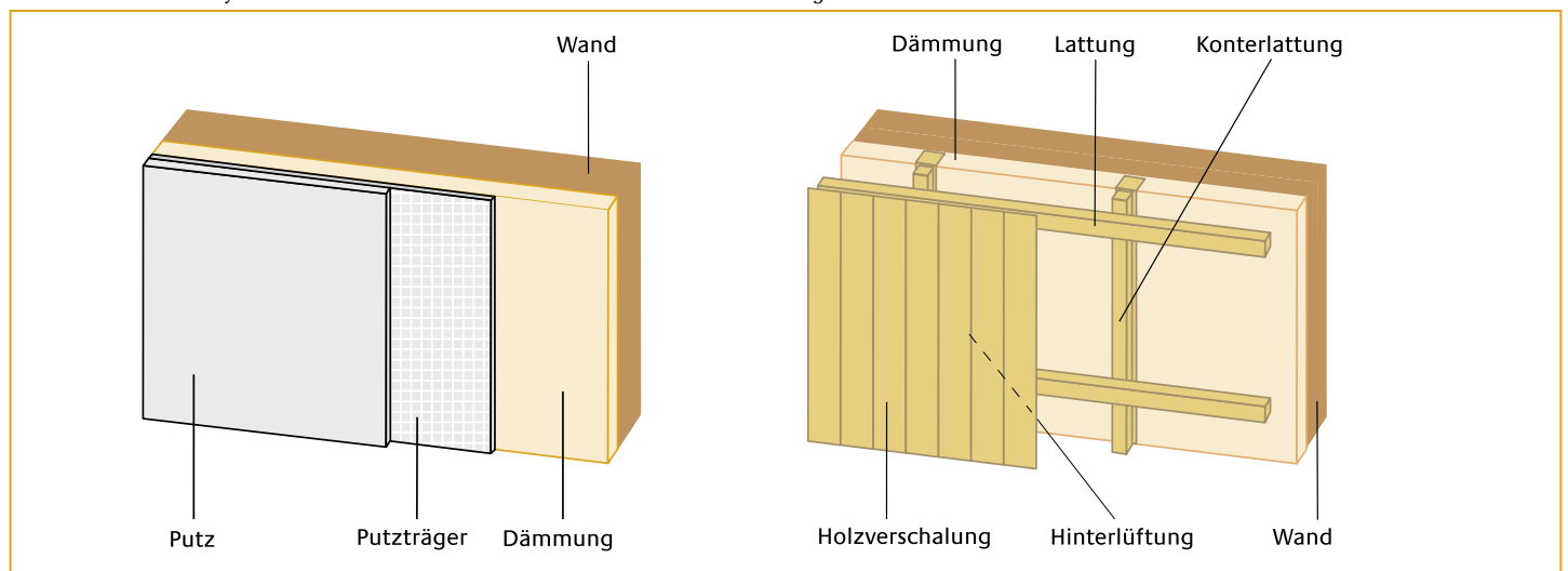
Wärmedämmverbundsystem
