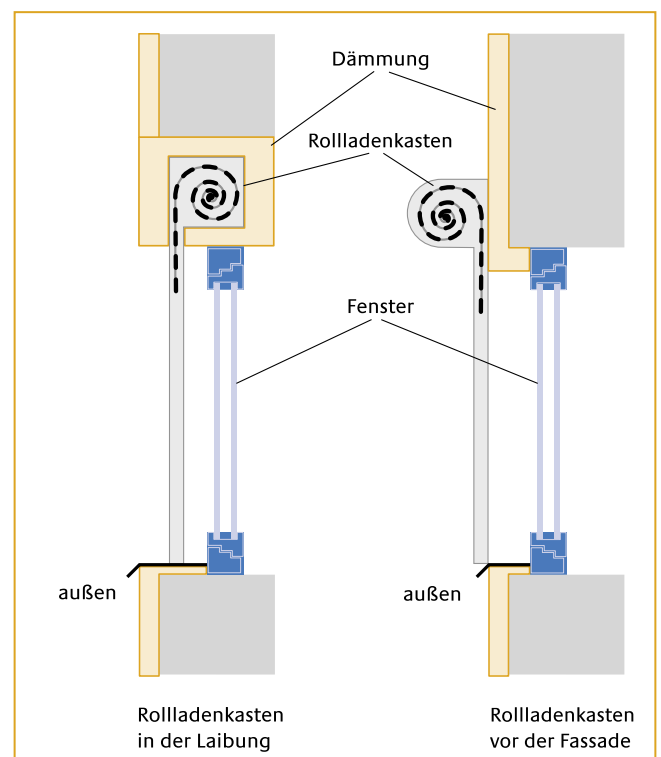
Rollladenkästen
