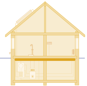
Dämmung Kellerdecke
