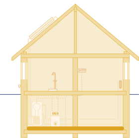
Dämmung Kellerfußboden
