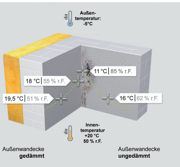
Oberflächentemperaturen [°C] und Luftfeuchte [%] der Innenseite einer Außenwand bei gedämmter und ungedämmter Außenwand
