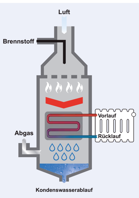
02 Brennwertheizung
