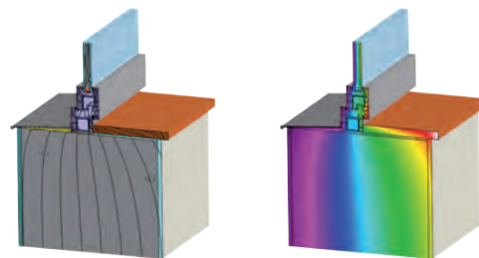
Fensteranschluss – ungedämmte Wand (Mauerwerk, Innen-/Außenputz)
